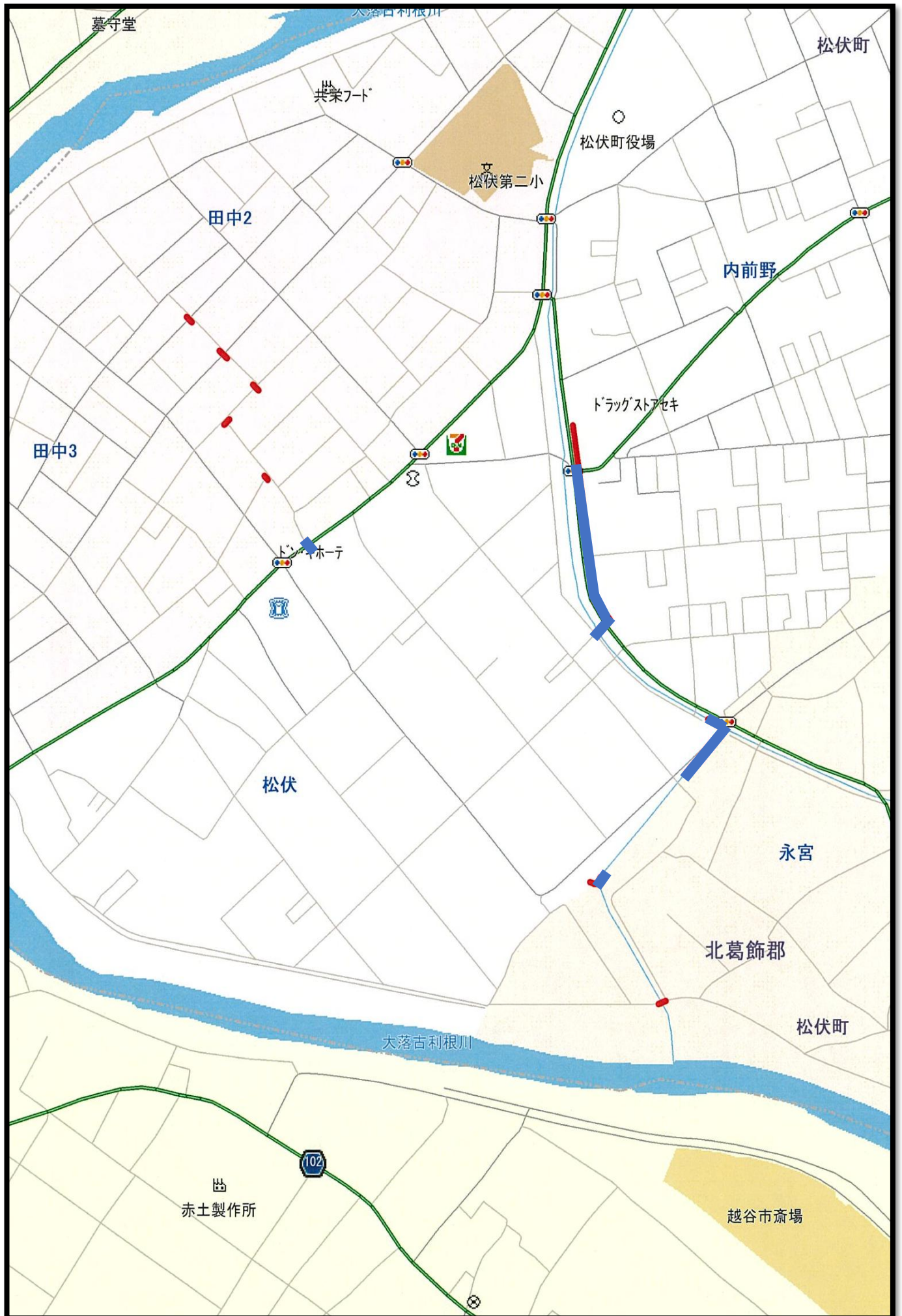
対応が必要とされる管路延長： ■ の箇所 0.85km(雨水管)
