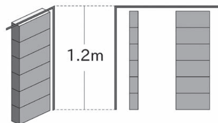
ブロック塀（高さの目安） 1.2mを超えると控え壁が必要
