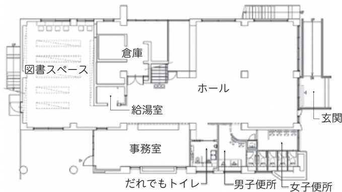
<多世代交流学習館 1階平面図>
